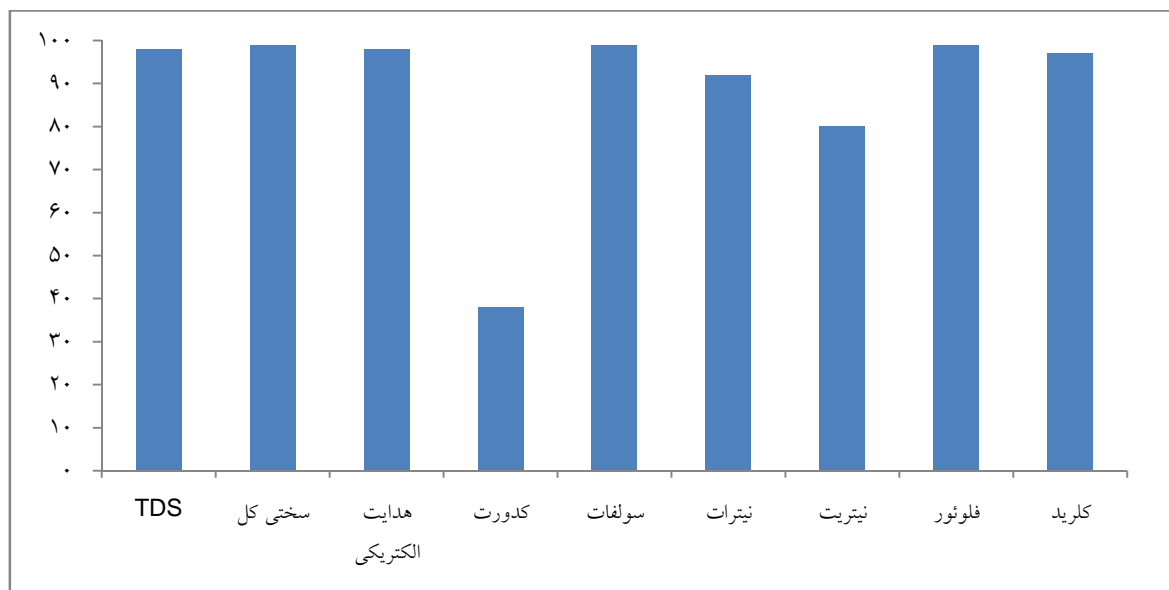
نمودار ۱. درصد راندمان حذف پارامترهای شیمیایی و فیزیکی آب ورودی و خروجی از دستگاه‌های آب شیرین‌کن قشم با استفاده از فرایندهای (Reverse Osmosis) RO
