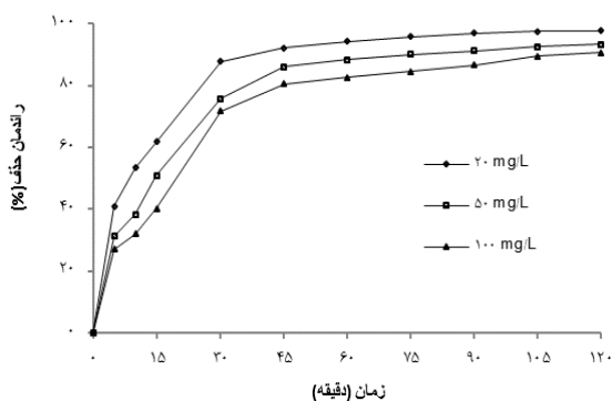
شکل ۴: تأثیر زمان تماس بروی کارایی حذف رنگ ( pH=5 ) و مقدار اولیه جاذب (۰/۵ گرم در ۵۰ میلی لیتر)
