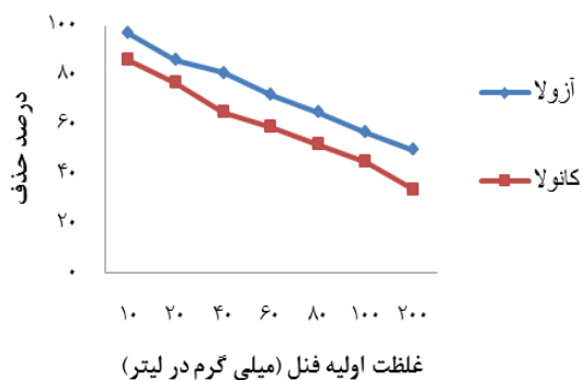
نمودار ۵: تأثیر غلظت اولیه فنل بر روی کارایی حذف (دوز جاذب ۱۰ g/l، زمان تماس ۹۰ و ۱۲۰ دقیقه، pH=۳)
