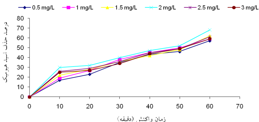
شکل ۵: تأثیر غلظت کیتوزان در فرآیند الکتروکواکولاسیون (pH=۶، غلظت اولیه اسید هیومیک ۵ mg/l، ولتاژ ۴۰ V)
