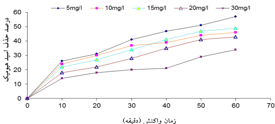
شکل ۴: تأثیر غلظت اولیه اسید هیومیک در فرآیند الکتروکواکولاسیون (بدون کیتوزان، ولتاژ ۴۰ V، pH=۶)
