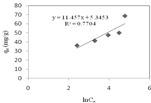
نمودار ۶: جذب سطحی رنگ ژانوس گرین توسط نانولوله کربنی چند دیواره بر اساس مدل جذب تمکین
