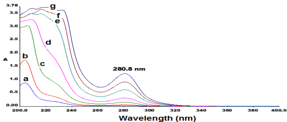
شکل ۱: طیف اسپکتروفوتومتری نالترکسون در غلظت‌های (a) ۰٫۱۰، (b) ۰٫۲۰، (c) ۰٫۵۰، (d) ۱٫۰۰، (e) ۲٫۰۰، (f) ۳۰۰ و (g) ۴۰۰ میکروگرم بر میلی‌لیتر
